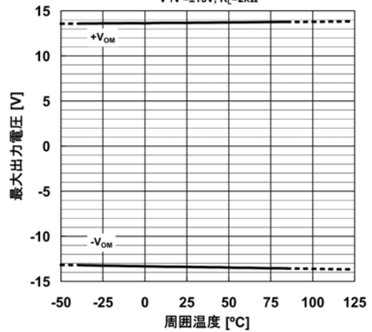
最大出力電圧 対 周囲温度 特性例 V + /V - =±15V, R L =2kΩ
