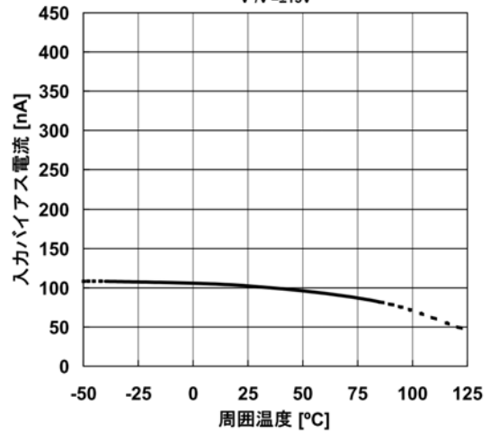
入力バイアス電流 対 周囲温度 特性例 V + /V - =±15V
