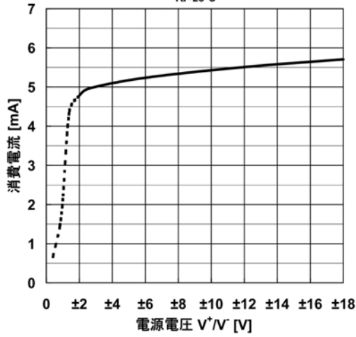
消費電流 対 電源電圧 特性例 Ta=25°C
