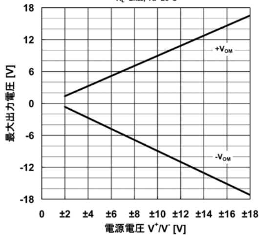
最大出力電圧 対 電源電圧 特性例 R L =2kΩ, Ta=25°C
